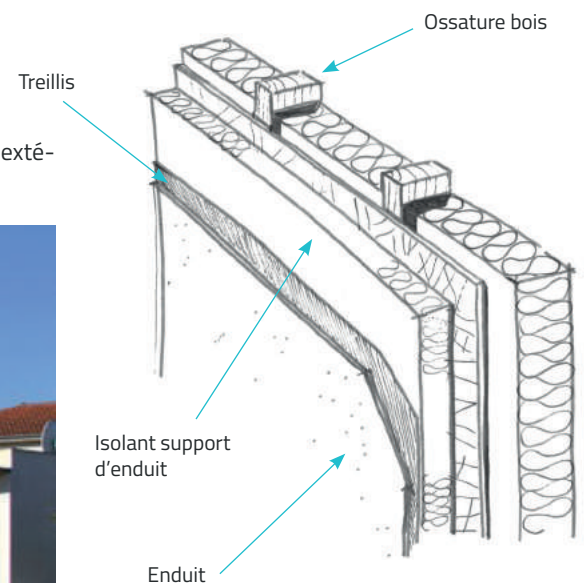
Ossature bois avec enduit sur panneau isolant.
