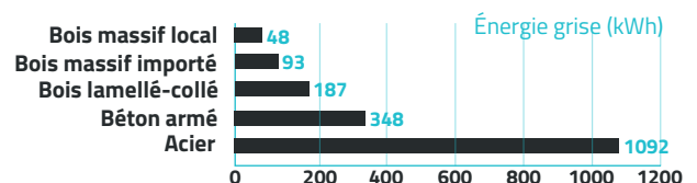
ÉNERGIE NÉCESSAIRE POUR LA FABRICATION DE DIFFÉRENTS MATÉRIAUX (pour une poutre de 3 mètres supportant 3 tonnes)
