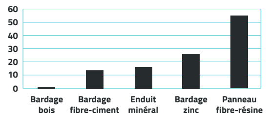
RÉCHAUFFEMENT CLIMATIQUE (KG CO 2 ÉQ. / M 2 )
